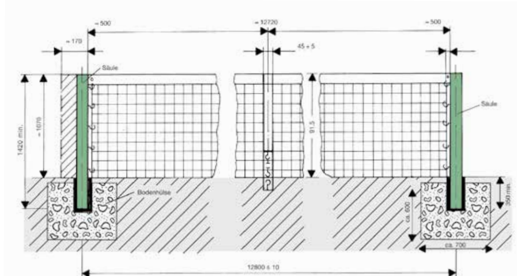
PFOSTEN- UND NETZABMESSUNG
