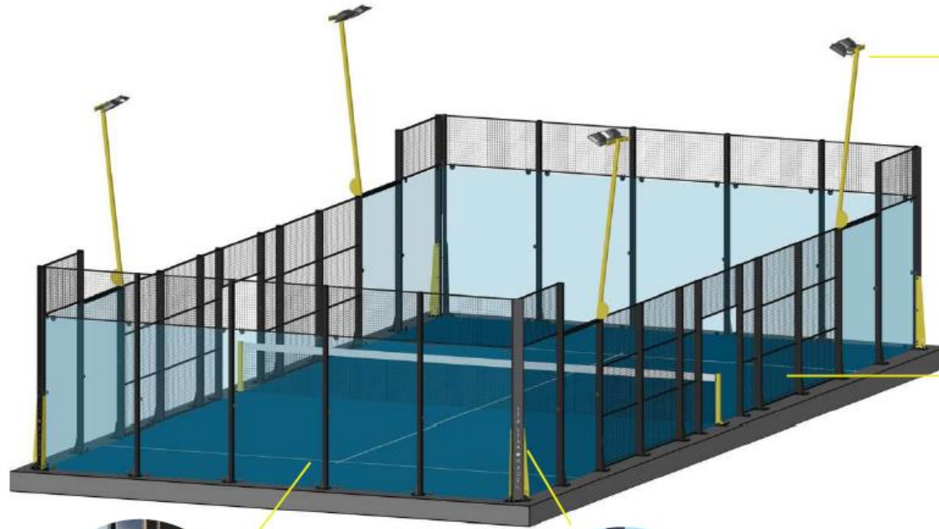
LED- und Blendschutz-Beleuchtung
