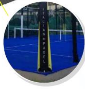
Stützpfosten mit Verstärkungsrippen, die mithilfe von 12 M16-Dübeln im Boden befestigt werden
